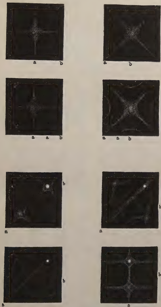
Fig. 217. CHLADNI FIGURES.*
